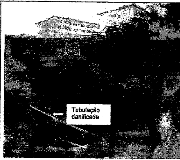
Fig.12 – Lançamento da estação Recanto dos Pássaros, tubo quebrado pela obra.
