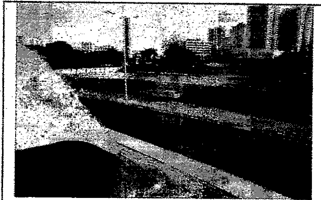
Fig.16 – Vista da parte superior da tubulação de 1000mm conduto forçado, com uma construção irregular sobre a mesma.
